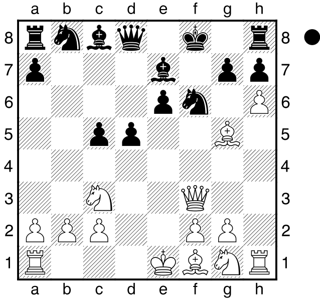
17.Bxd7 Diagram
